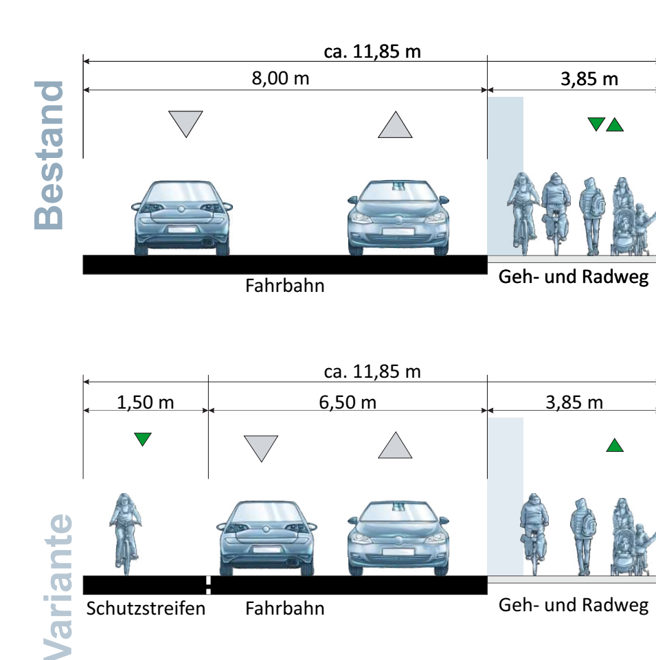
Querschnitt B202
