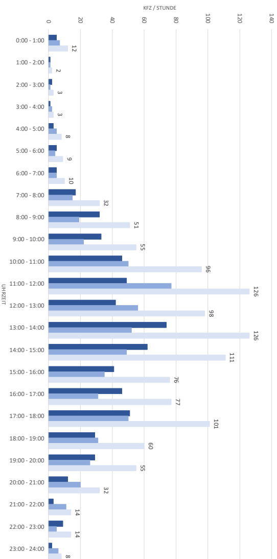
Tagesganglinie (alle Kfz, Querschnitt und richtungsgetrennt)
