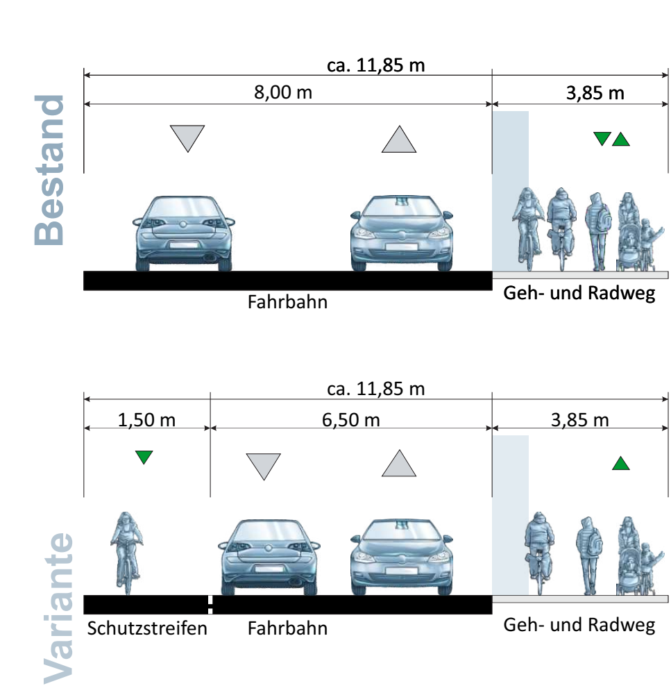
Querschnitt B202
